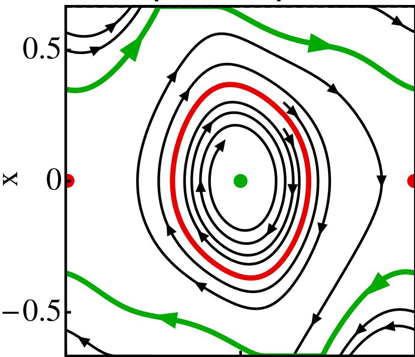
puller( p < 0 )
