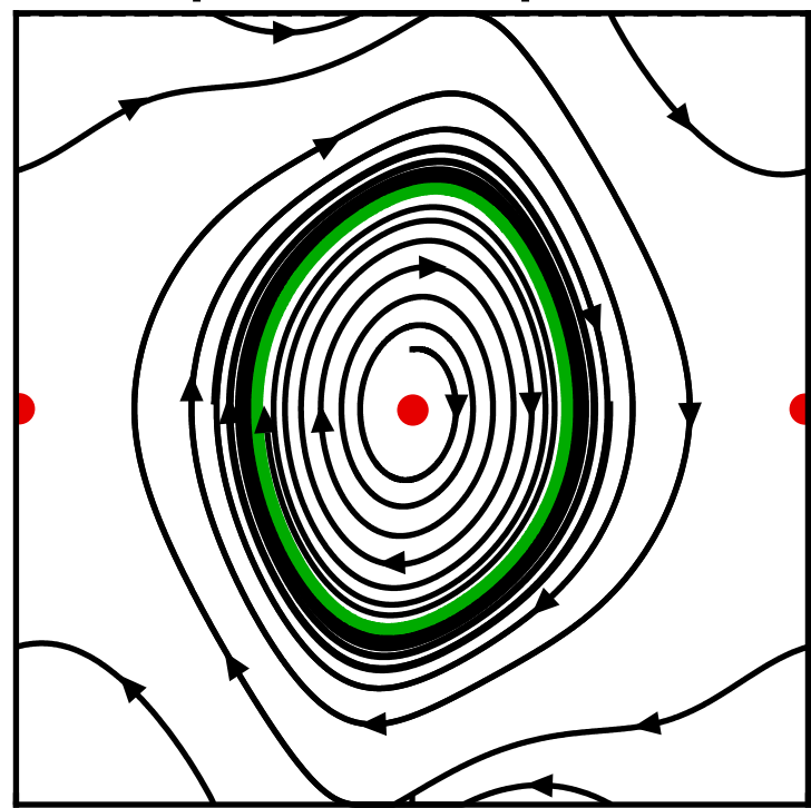
pusher( p > 0 )
