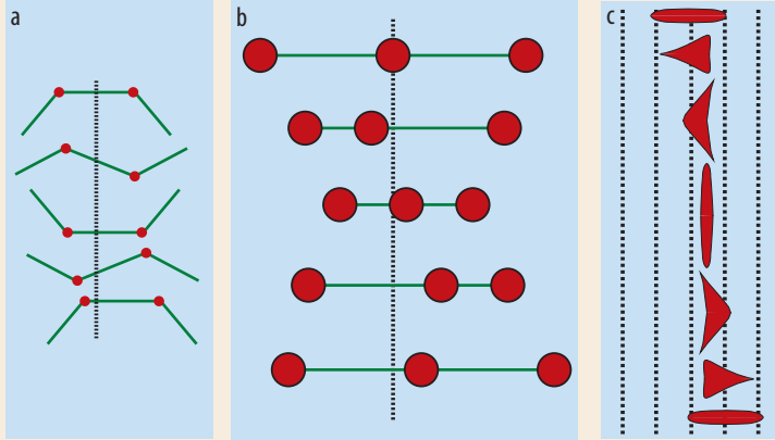
Abb. 1 Verschiedene Schwimmer mit nicht-reziproker periodischer Schlagbewegung: Beim Purcell-Schwimmer (a) bewegen sich die beiden äußeren Elemente abwechselnd nach oben oder unten, wobei das jeweils andere Gelenk fest bleibt. Beim linearen Drei-Kugel-Schwimmer (b) bewegen sich die beiden äußeren Kugeln abwechselnd auf die mittlere
